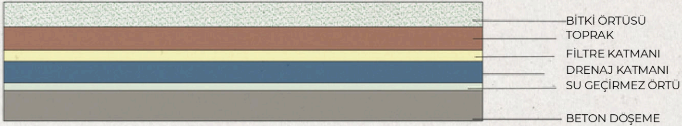
YEŞİL ÇATI KESİTİ
