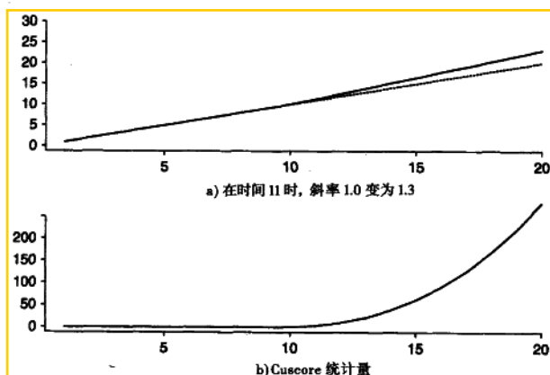
图 11-6 趋势变化的识别
