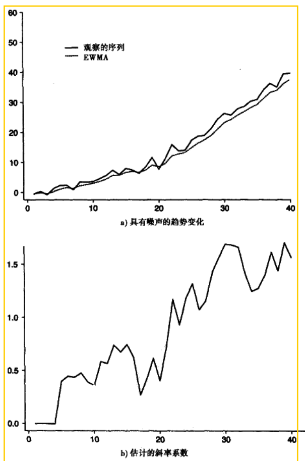
图 11-14 噪声影响下的斜率系数估计值 \beta_t = 0.25(EWMA_t - EWMA_{t-4})
