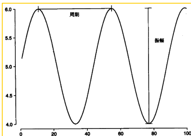
图 9-2 正弦波
