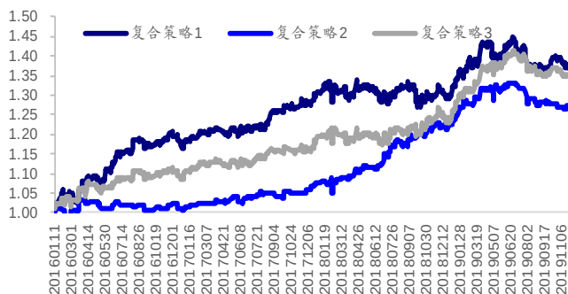
图37 IH 精细化回测净值
