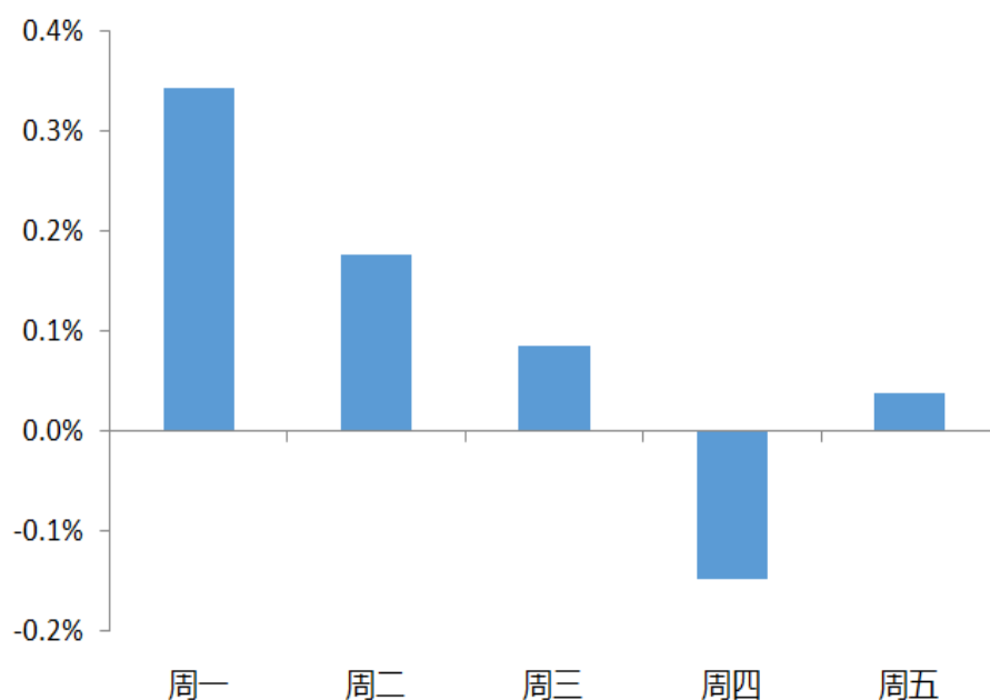
图 2：涨跌幅的周内效应（全部 A 股）
