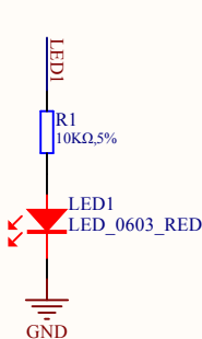
状态指示灯
