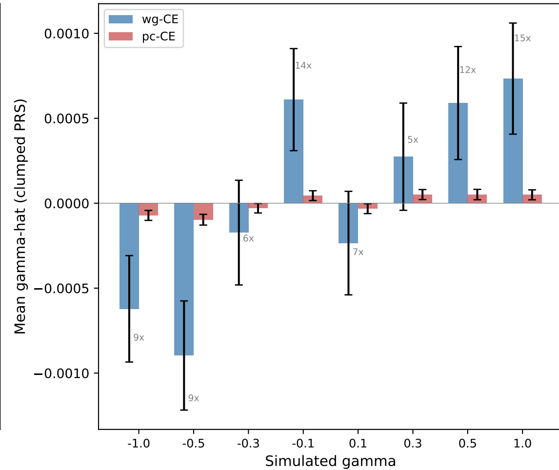
C. wg-CE vs pc-CE gamma-hat
