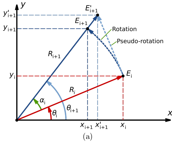
Figura 9: (a) Rotação do vetor, relativo ao sistema ortogonal, e (b) rotação do sistema de coordenadas.
