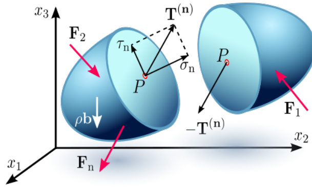
Figura 10: Força interna resultante \mathbf{T}^{(n)} de uma seção com orientação arbitrária.
