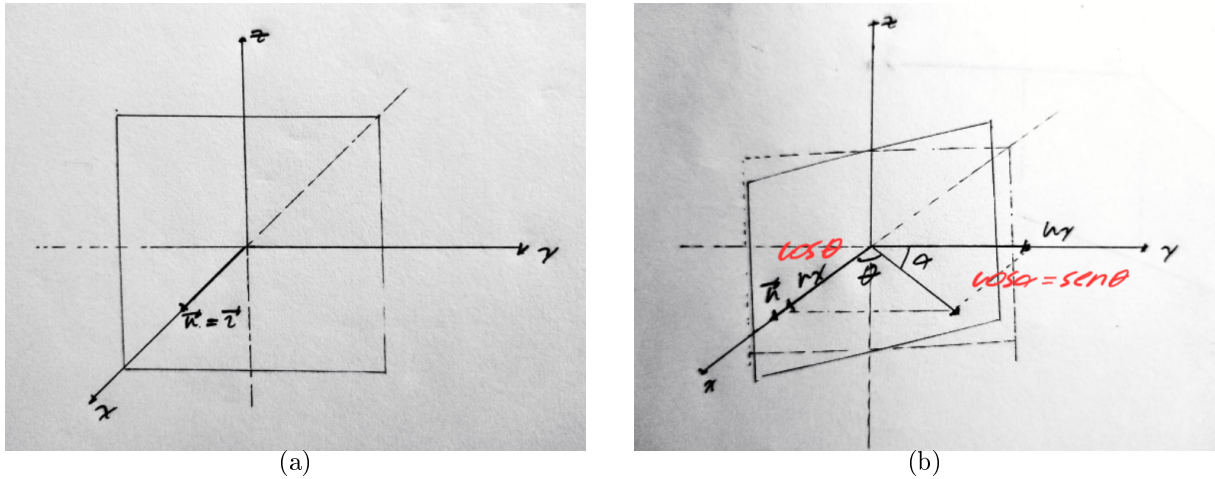
Figura 7: (a) Tensões no sistema resultante sob rotação e (b) a relação de projeção entre as tensões dos dois sistemas.
