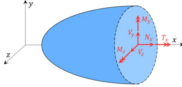
Figura 11: Estado de tensão em um plano perpendicular ao eixo x do sistema cartesiano.
