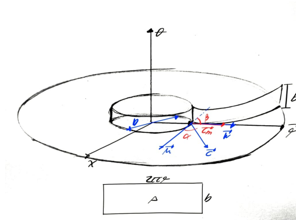
Figura 13: Área da seção transversal do rotor perpendicular à componente \vec{c}_m , em regime de escoamento radial.
