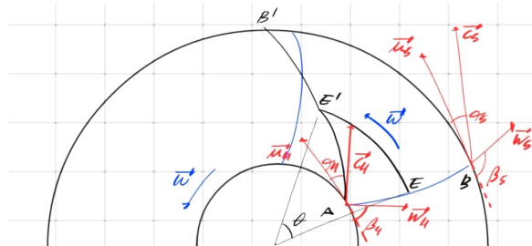
Figura 9: Velocidade tangencial \vec{u} , o qual descreve uma circunferência de raio \vec{r} .
