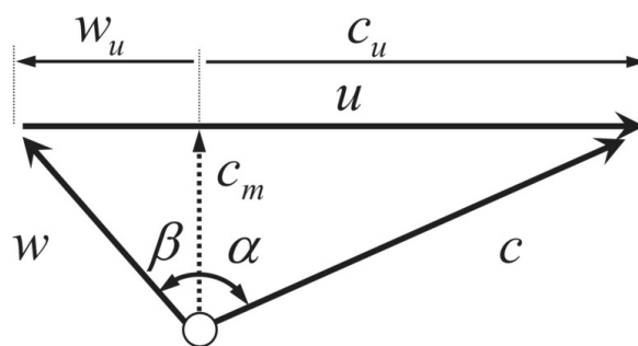
Figura 12: Triângulo de velocidades de uma máquina de fluxo, segundo a Eq. 7.
