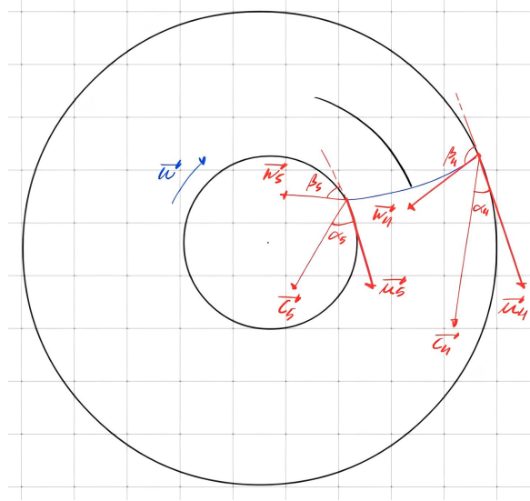
Figura 11: Velocidade tangencial \vec{u} , o qual descreve uma circunferência de raio \vec{r} .
