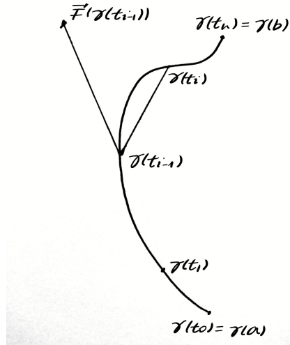
Figura 5: Força \vec{F}(\gamma(t_{i-1})) aplicada a uma distância infinitesimal \gamma(t_i) - \gamma(t_{i-1}) .
