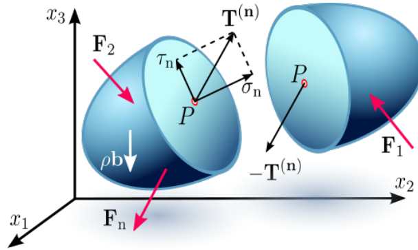
Figura 9: Força interna resultante \mathbf{T}^{(n)} de uma seção com orientação arbitrária.
