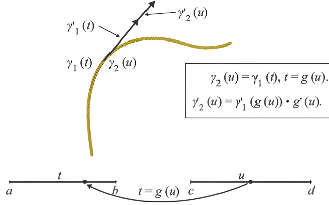
Figura 7: Vetor tangente às curvas \gamma_1(t) e \gamma_2(u) no ponto t = g(u) .
