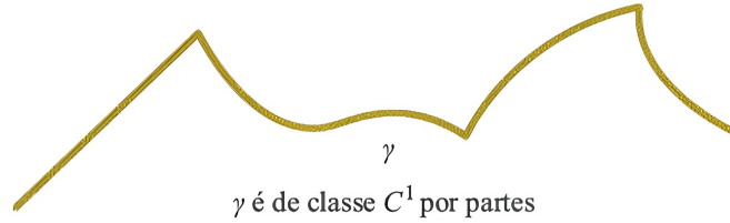
Figura 6: Curva \gamma por partes.
