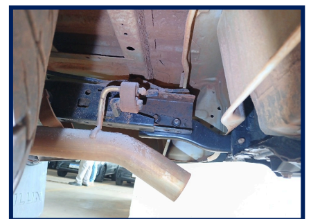
Longarina traseira/esquerda
