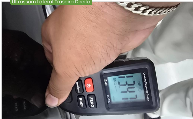
Ultrassom Lateral Traseira Direita
