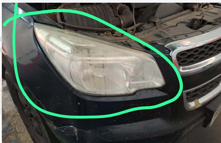
Farol com excesso de umidade
