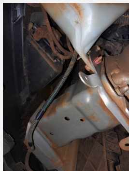
LONGARINA DIANTEIRA ESQUERDA
