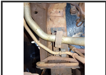
LONGARINA DIANTEIRA DIREITA
