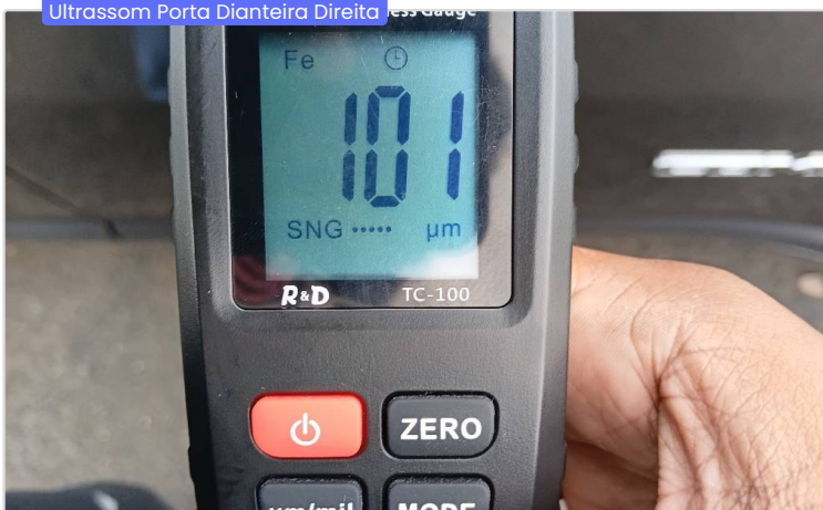
Ultrassom Porta Dianteira Direita
