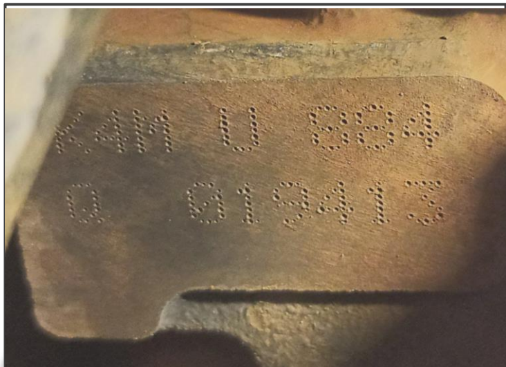
Foto do Número do Motor: K4MU884Q019413
