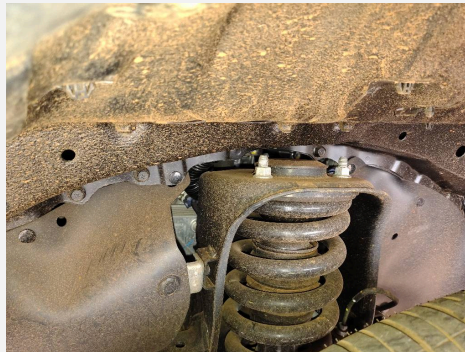
TORRE DO AMORTECEDOR ESQUERDA
