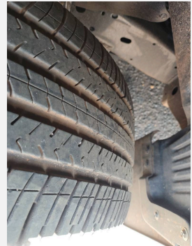
PDE
