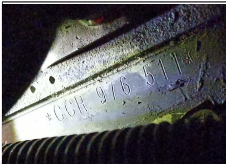
Foto do Número do Motor: CCR976511
