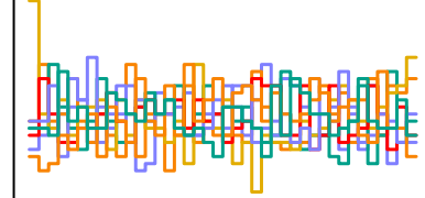
a_sent[281] n_eff = 5158
