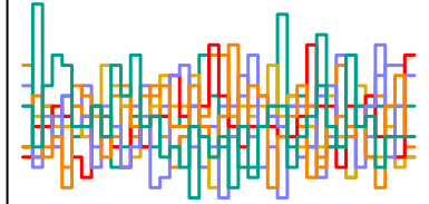
b_auth[9] n_eff = 3063
