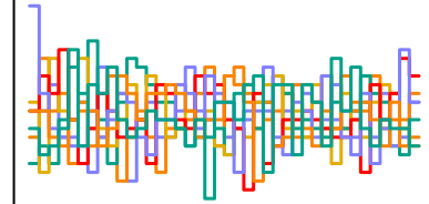
z_sent[42] n_eff = 7022
