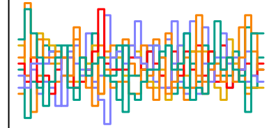
delta_j_th[2] n_eff = 5136
