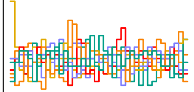
a_sent[57] n_eff = 5456
