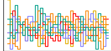
a_sent[158] n_eff = 5234
