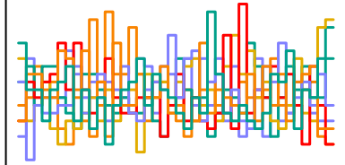
delta_j_pos[3] n_eff = 5905
