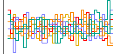
z_dia[2] n_eff = 2777
