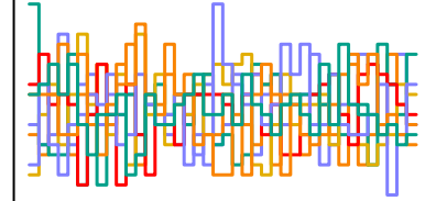
b_auth[11] n_eff = 2458
