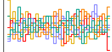
a_sent[56] n_eff = 2063
