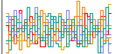
a_sent[177] n_eff = 5118
