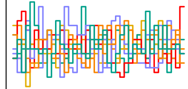
b_auth[5] n_eff = 4113
