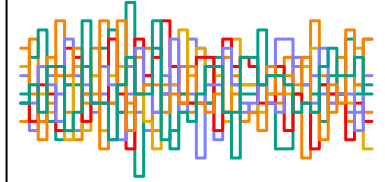
z_sent[292] n_eff = 7628
