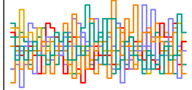
a_sent[277] n_eff = 4300
