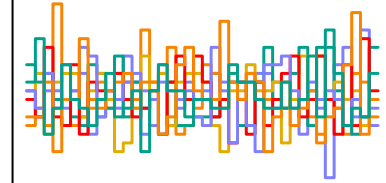
b_auth[8] n_eff = 6369
