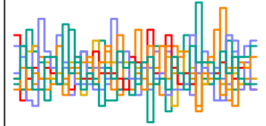
b_auth[10] n_eff = 5674
