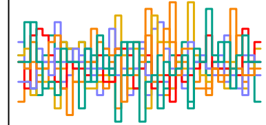
b_auth[2] n_eff = 4286
