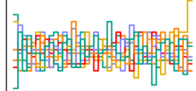
a_sent[275] n_eff = 4315
