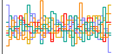
a_sent[265] n_eff = 3066
