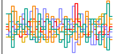
delta_j_th[3] n_eff = 5136
