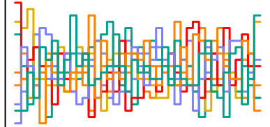
a_sent[232] n_eff = 2735
