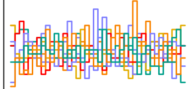
a_sent[94] n_eff = 5526
