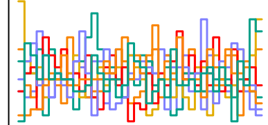
a_sent[23] n_eff = 5011
