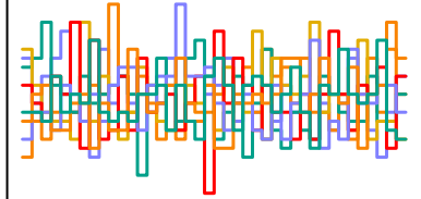
b_auth[7] n_eff = 2160
