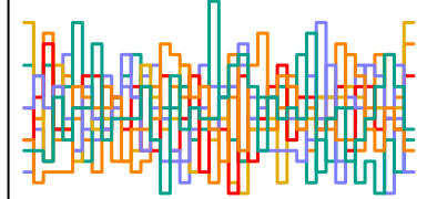
a_sent[49] n_eff = 5190
