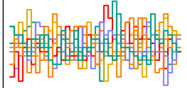
d_adj n_eff = 4427
