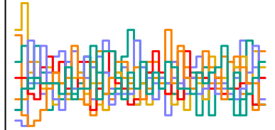
a_sent[223] n_eff = 3019
