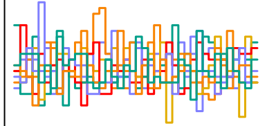
b_auth[1] n_eff = 3320
