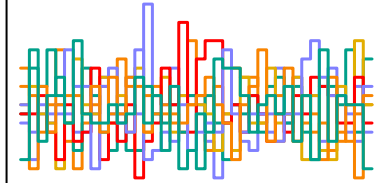
b_auth[4] n_eff = 3613
