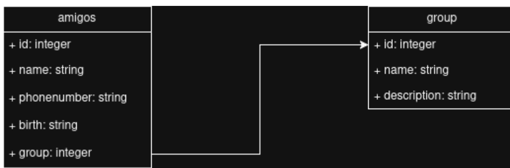
Figura 1. Modelagem do banco de dados
