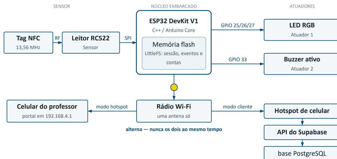
Figura 1 — Diagrama de blocos. A API encena o papel do sistema acadêmico da UVA, ao qual não temos acesso: é dela que vem a lista da turma e é para ela que vai o relatório.
