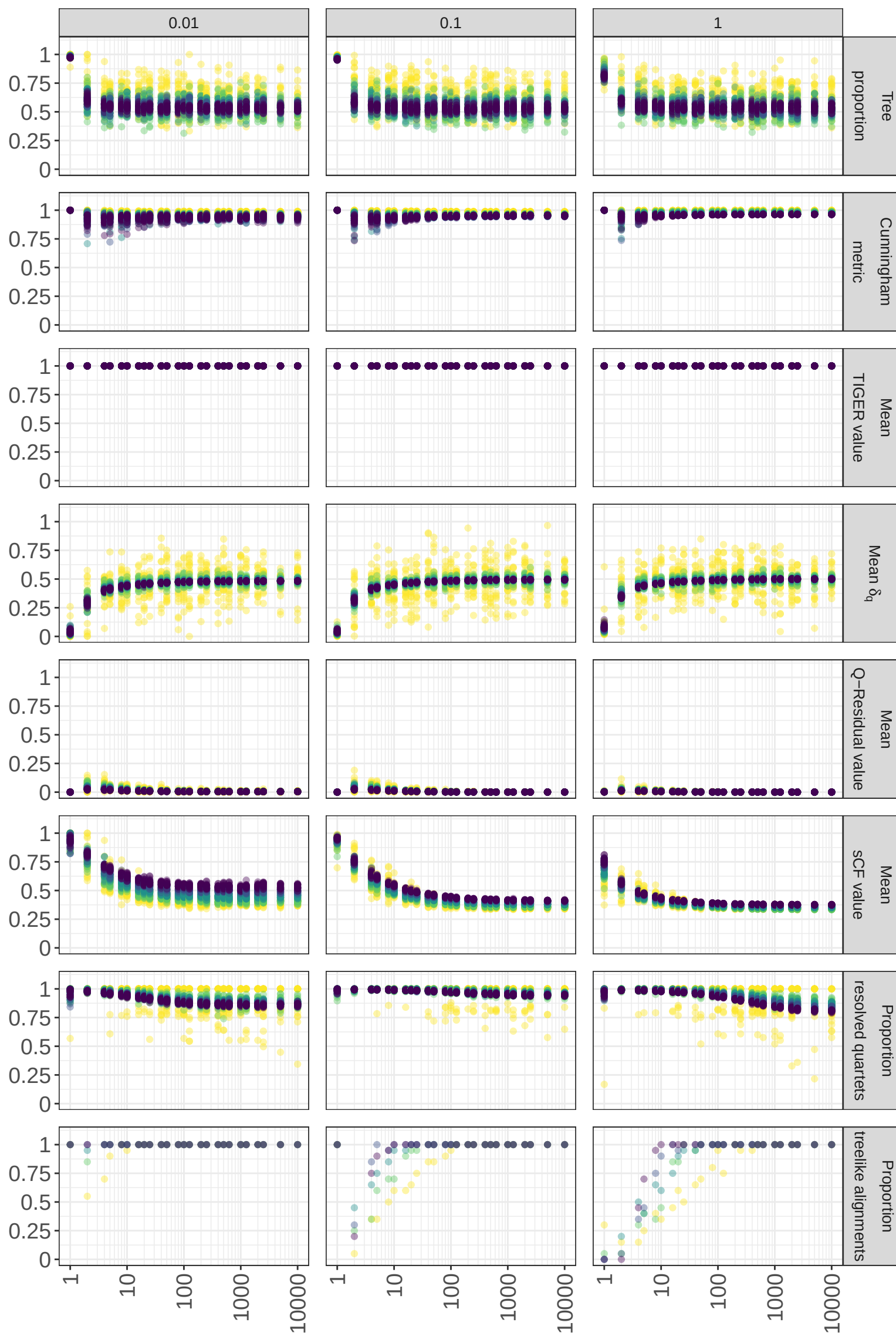
Tree depth (Rescaled trees) (substitutions per site)
