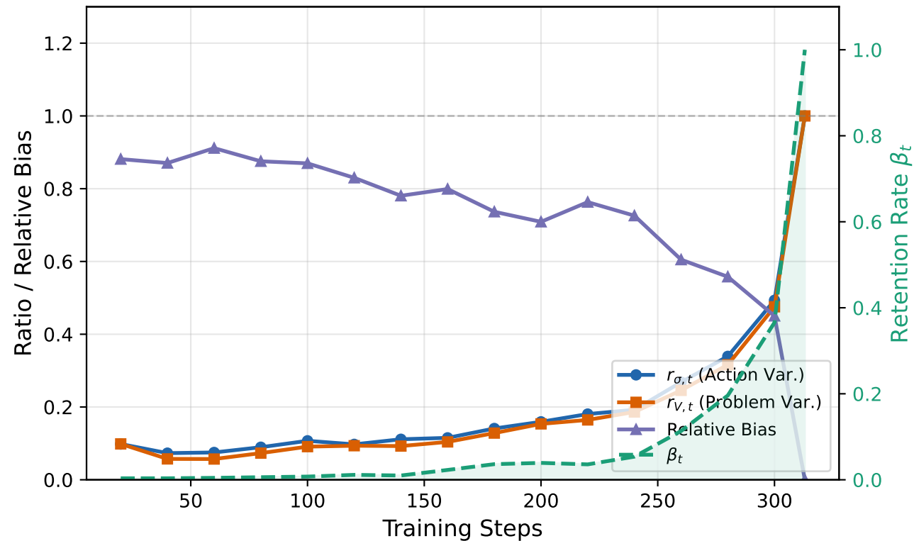
Llama-3.2-3B (Oracle)
