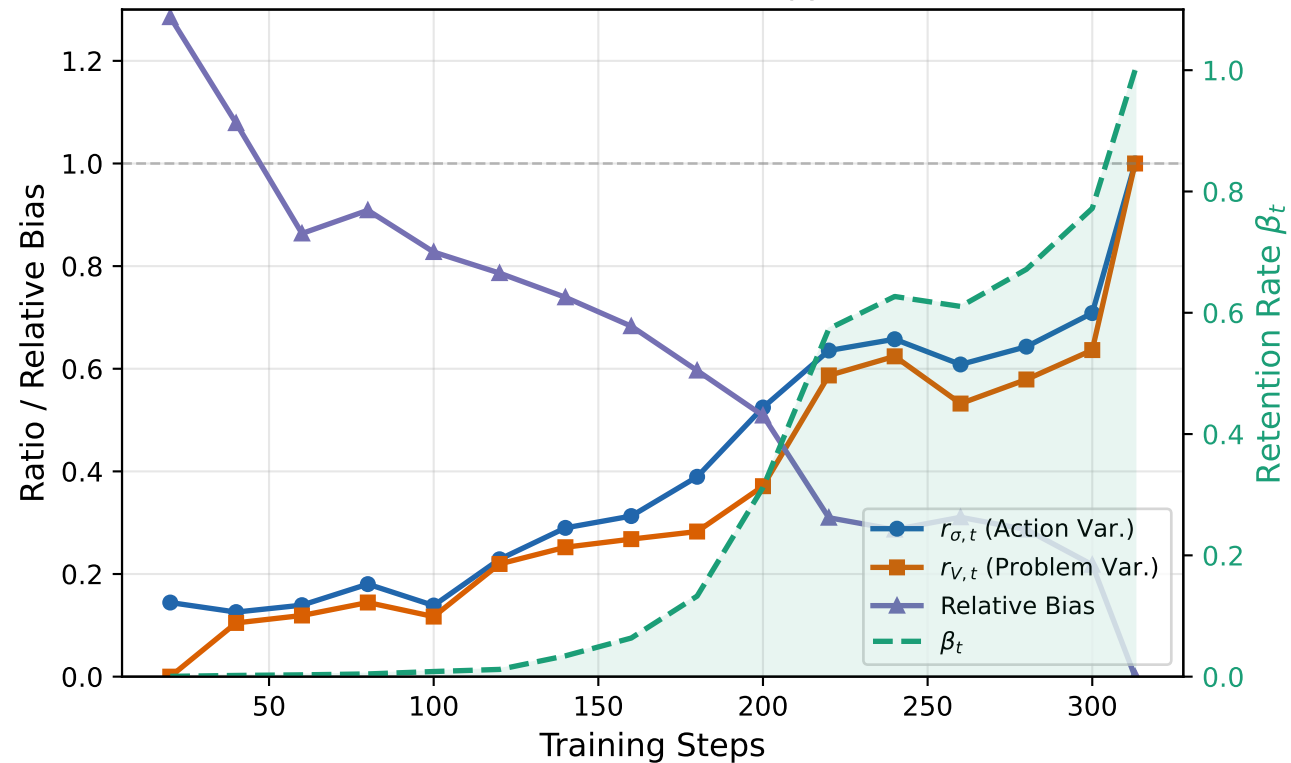
Llama-3.2-3B (Entropy)
