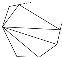
FIGURE 8-23. n -gon ( n-2 triangles).
