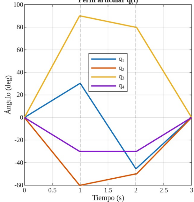
Perfil articular q(t)
