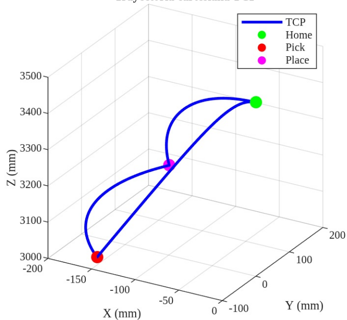
Trayectoria cartesiana TCP
