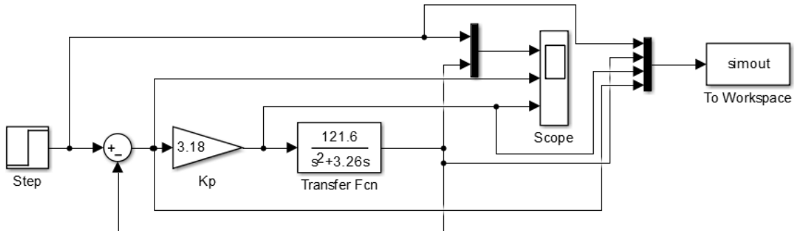
Figura 5: Diagrama para simulación del sistema en lazo cerrado con K_p = 3.18 para r = \pi [rad] en simulink.
