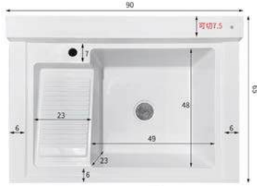
MODEL NUMBER 90×65 单盆带搓 单位: cm 外径: 90×65 颜色: 珠光白, 高级灰, 高级黑 银星白, 浅灰, 卡其, 可丽耐
