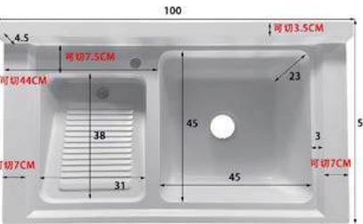
MODEL NUMBER 100×58 双盆带搓 单位: cm 外径: 100×58 颜色: 珠光白, 高级灰, 高级黑 银星白, 浅灰, 卡其, 可丽耐
