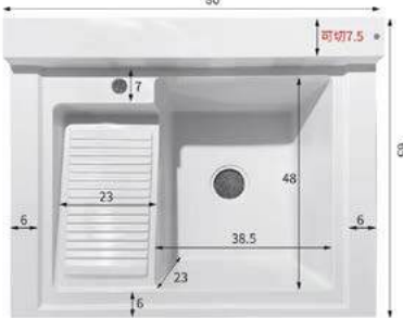
MODEL NUMBER 80×65 单盆带搓 单位: cm 外径: 80×65 颜色: 珠光白, 高级灰, 高级黑 银星白, 浅灰, 卡其, 可丽耐
