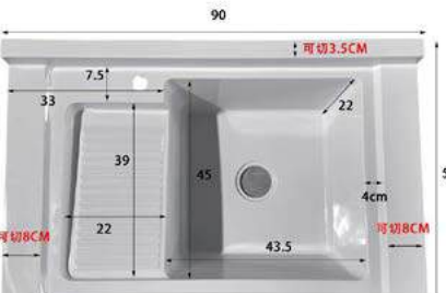
MODEL NUMBER 90×58 单盆带搓 单位: cm 外径: 90×58 颜色: 珠光白, 高级灰, 高级黑 银星白, 浅灰, 卡其, 可丽耐
