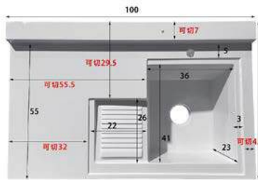
MODEL NUMBER 100×63 带搓右盆左切角 单位: cm 外径: 100×63 颜色: 珠光白, 高级灰, 高级黑 银星白, 浅灰, 卡其, 可丽耐
