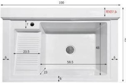
MODEL NUMBER 100×65 单盆带搓 单位: cm 外径: 100×65 颜色: 珠光白, 高级灰, 高级黑 银星白, 浅灰, 卡其, 可丽耐
