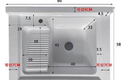
MODEL NUMBER 80×58 单盆带搓 单位: cm 外径: 80×58 颜色: 珠光白, 高级灰, 高级黑 银星白, 浅灰, 卡其, 可丽耐
