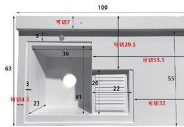
MODEL NUMBER 100×63 带搓左盆右切角 单位: cm 外径: 100×63 颜色: 珠光白, 高级灰, 高级黑 银星白, 浅灰, 卡其, 可丽耐
