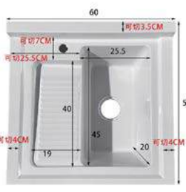
MODEL NUMBER 60×58 单盆带搓 单位: cm 外径: 60×58 颜色: 珠光白, 高级灰, 高级黑 银星白, 浅灰, 卡其, 可丽耐
