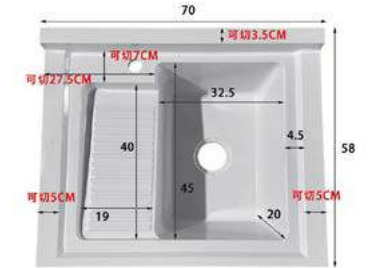
MODEL NUMBER 70×58 单盆带搓 单位: cm 外径: 70×58 颜色: 珠光白, 高级灰, 高级黑 银星白, 浅灰, 卡其, 可丽耐
