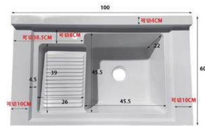
MODEL NUMBER 100×60 右单盆带搓 单位: cm 外径: 100×60 颜色: 珠光白, 高级灰, 高级黑 银星白, 浅灰, 卡其, 可丽耐
