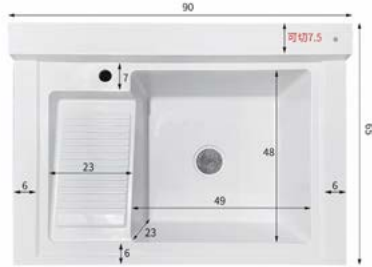
MODEL NUMBER 90×65 单盆带搓 单位: cm 外径: 90×65 颜色: 珠光白, 高级灰, 高级黑 银星白, 浅灰, 卡其, 可丽耐
