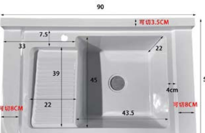
MODEL NUMBER 90×58 单盆带搓 单位: cm 外径: 90×58 颜色: 珠光白, 高级灰, 高级黑 银星白, 浅灰, 卡其, 可丽耐
