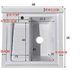
MODEL NUMBER 60×58 单盆带搓 单位: cm 外径: 60×58 颜色: 珠光白, 高级灰, 高级黑 银星白, 浅灰, 卡其, 可丽耐
