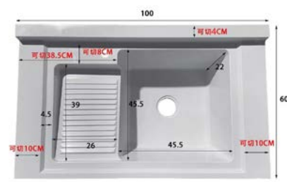
MODEL NUMBER 100×60 右单盆带搓 单位: cm 外径: 100×60 颜色: 珠光白, 高级灰, 高级黑 银星白, 浅灰, 卡其, 可丽耐
