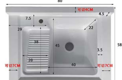
MODEL NUMBER 80×58 单盆带搓 单位: cm 外径: 80×58 颜色: 珠光白, 高级灰, 高级黑 银星白, 浅灰, 卡其, 可丽耐
