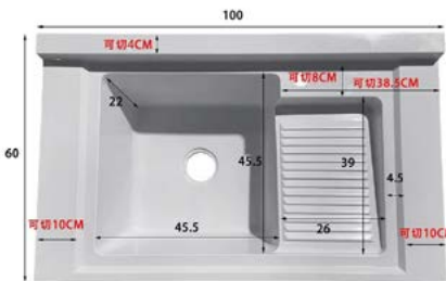
MODEL NUMBER 100×60 左单盆带搓 单位: cm 外径: 100×60 颜色: 珠光白, 高级灰, 高级黑 银星白, 浅灰, 卡其, 可丽耐
