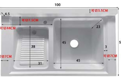
MODEL NUMBER 100×58 双盆带搓 单位: cm 外径: 100×58 颜色: 珠光白, 高级灰, 高级黑 银星白, 浅灰, 卡其, 可丽耐
