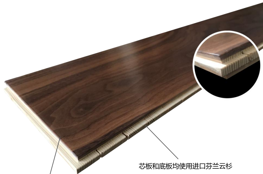
光益实木三层地板
