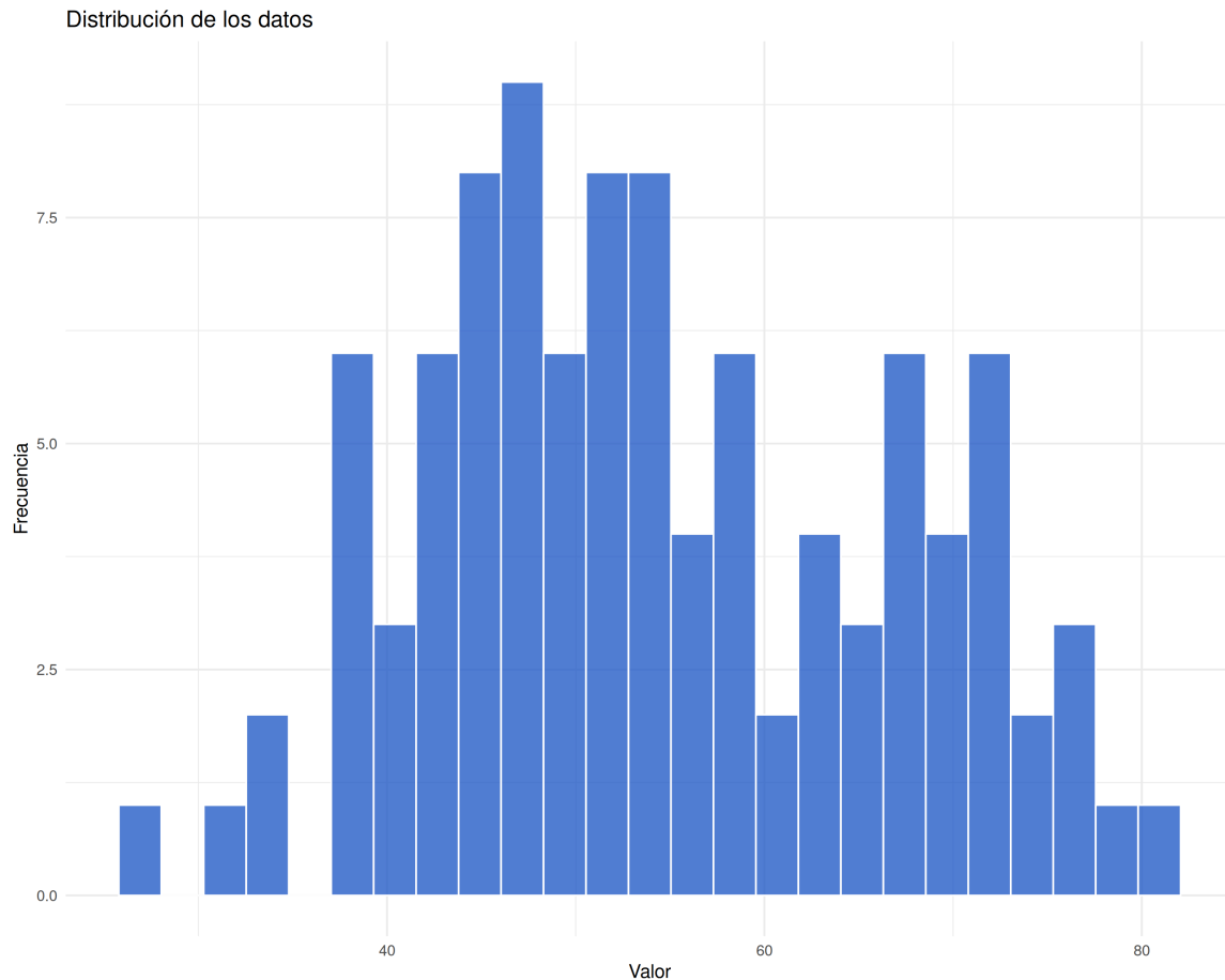
Figura 2: Histograma de los datos simulados
