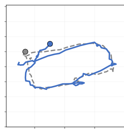
G2VLM
