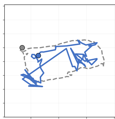
StreamVGGT
