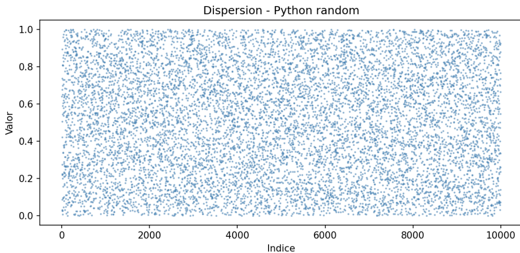
Figura 6: Gráfico de dispersión de valores generados mediante el generador random de Python.
