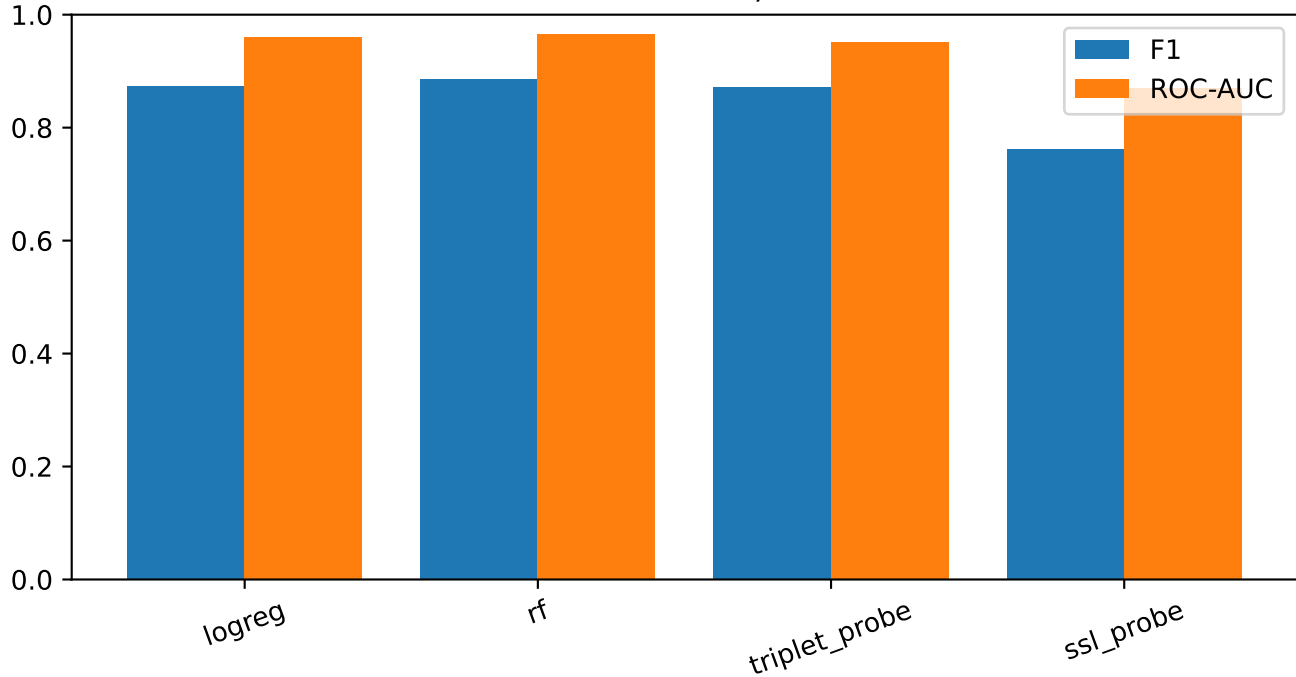
Classification — F1 / ROC-AUC
