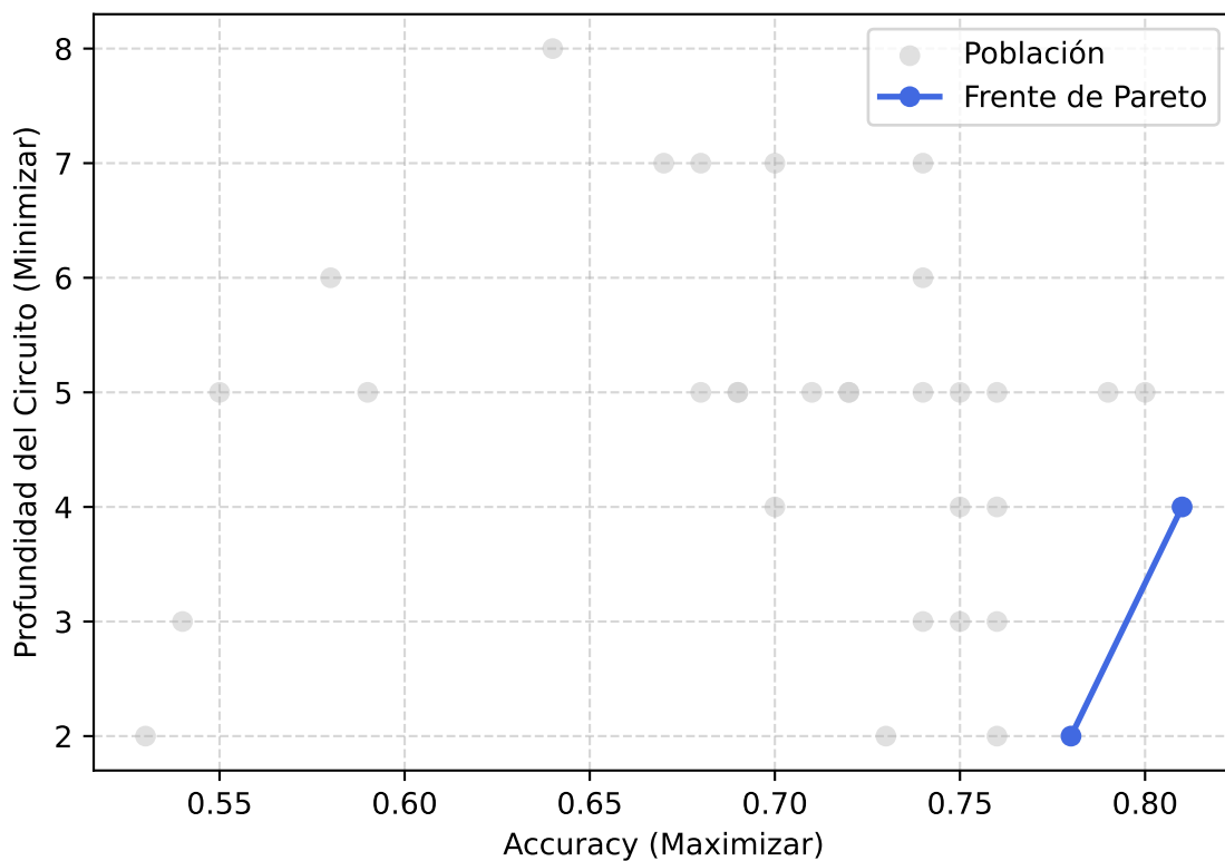
Generación 82
