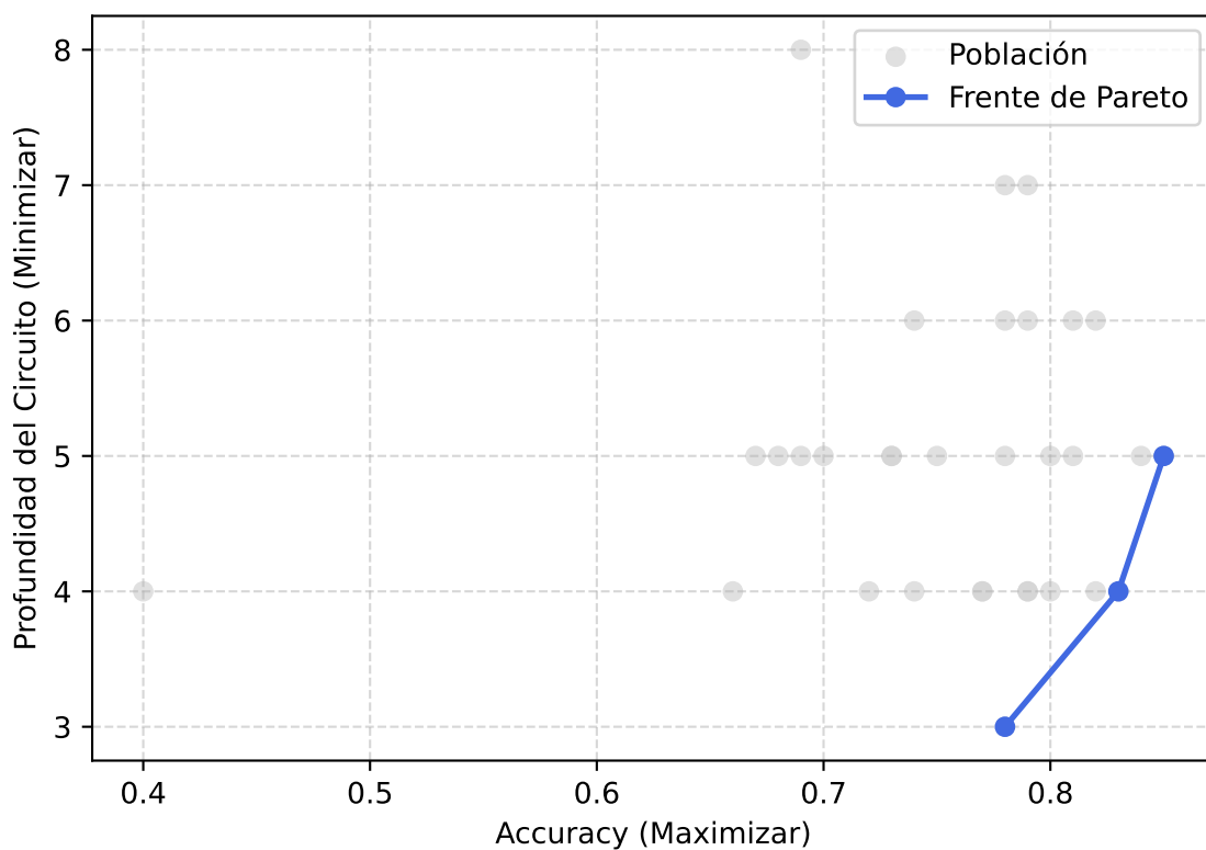
Generación 82
