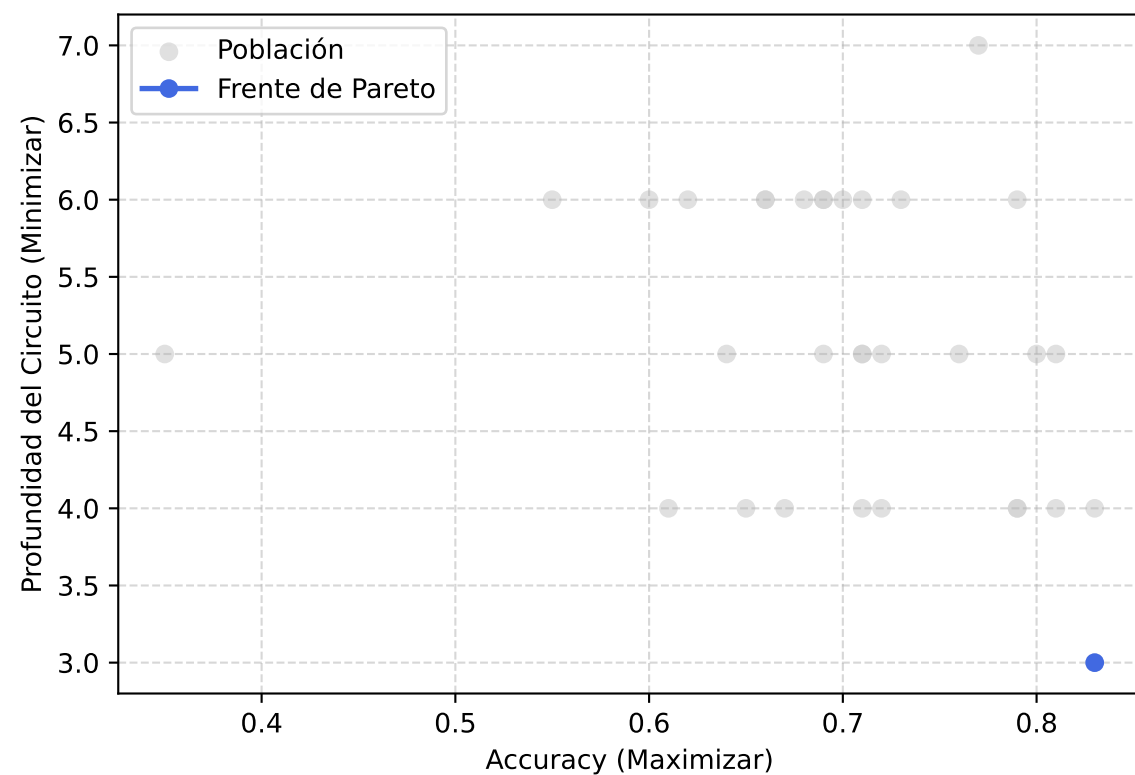
Generación 123
