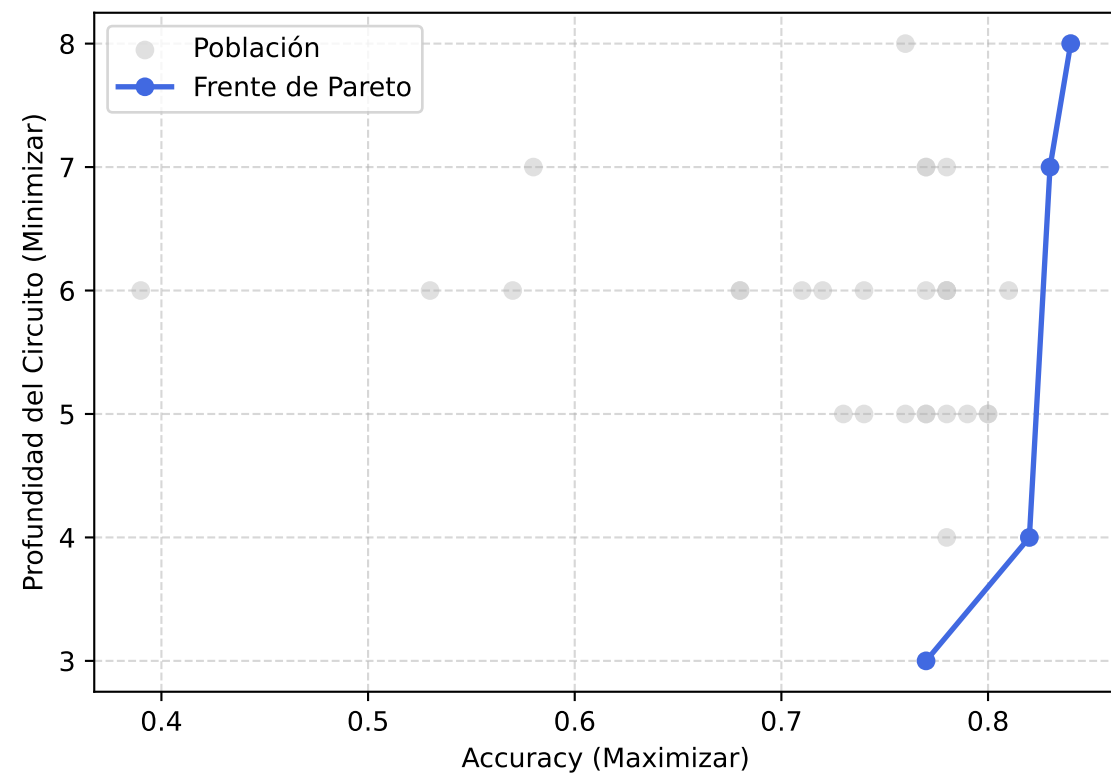
Generación 123
