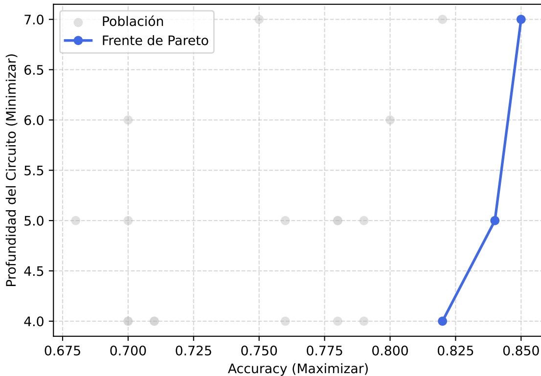
Generación 36
