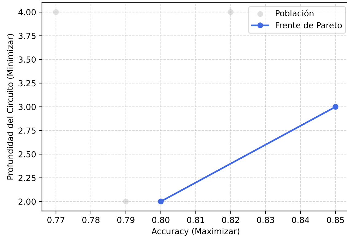
Generación 55
