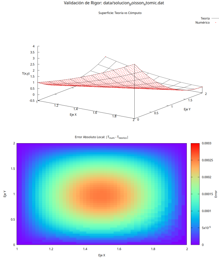
Figura 2: Solución numérica de la ecuación de Poisson 2D para una malla 50 \times 50 usando la implementación atomic .
