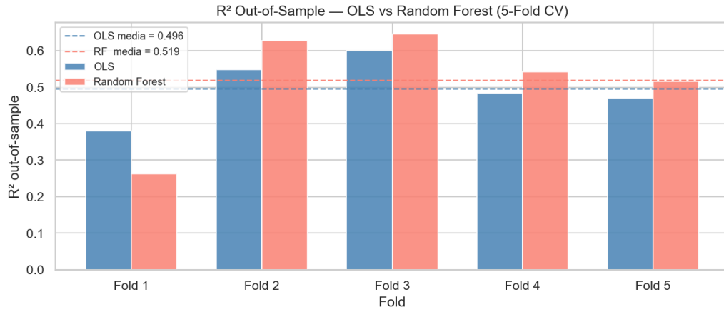
Figura 3.3: R^2 out-of-sample por fold en la validación cruzada de 5 folds para OLS y Random Forest. Las líneas punteadas indican los promedios (OLS: 0,496, RF: 0,519). La variabilidad entre folds es mayor en el RF, reflejo de su mayor sensibilidad a la composición de la muestra de training.
