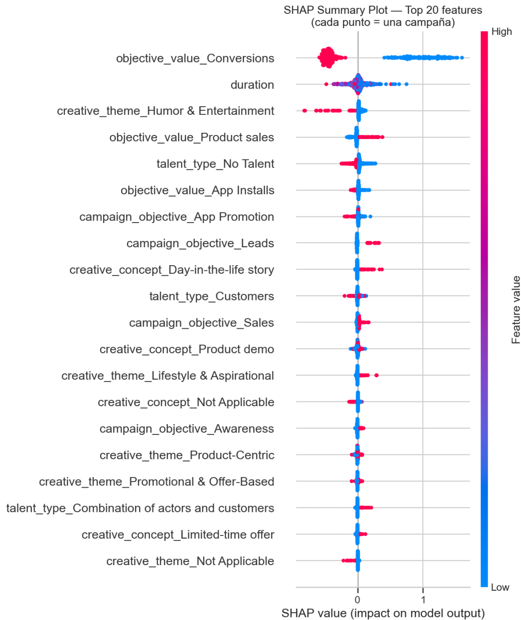
Figura 4.3: SHAP beeswarm plot : las 20 variables con mayor importancia promedio |\text{SHAP}| . Cada punto representa una observación. El color indica el valor de la variable (rojo = alto, azul = bajo). La posición horizontal indica el impacto en la predicción del modelo.
