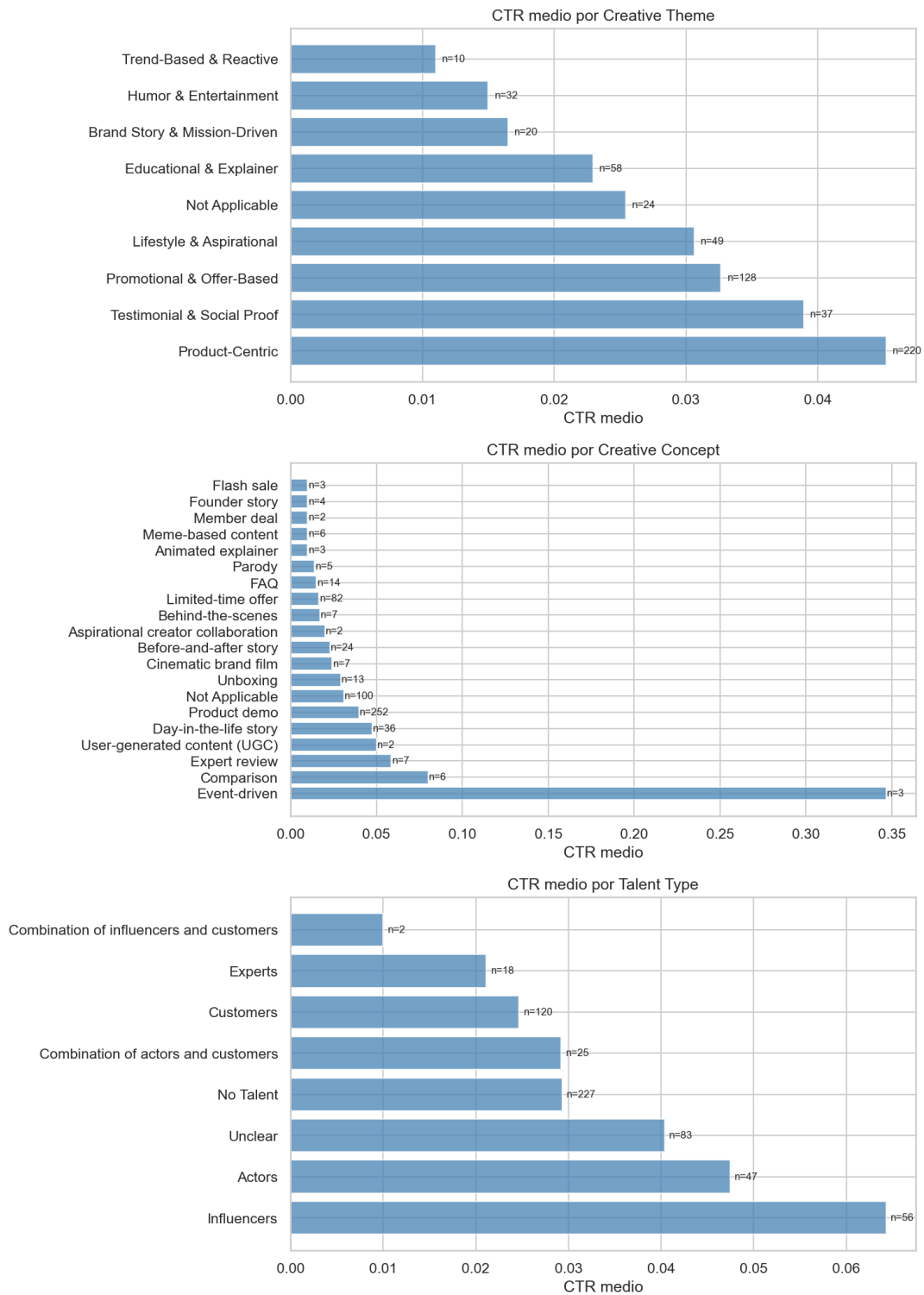
Figura 4.1: CTR medio por categoría para las tres dimensiones creativas analizadas. Las barras representan el CTR promedio por grupo. El tamaño de muestra por categoría varía considerablemente.
