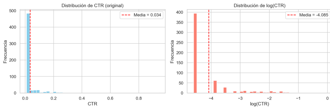
Figura 3.1: Distribución del CTR original (izquierda) y de \log(CTR) (derecha). La transformación logarítmica reduce la asimetría de 6,78 a 1,87 y elimina la cola derecha extrema, haciendo la distribución más apta para el modelo OLS. El pico visible en \log(CTR) \approx -4,6 corresponde al valor mínimo reportado de CTR = 0,01 ( floor effect ).
