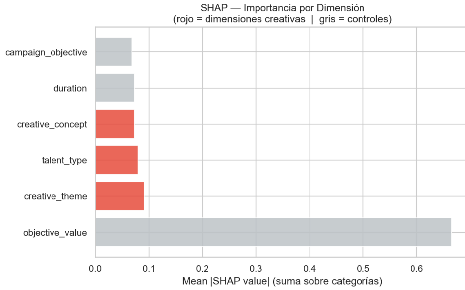
Figura 4.4: Importancia SHAP media ( |\text{SHAP}| ) agregada por dimensión creativa. Las barras representan la contribución promedio de cada dimensión a las predicciones del modelo Random Forest.
