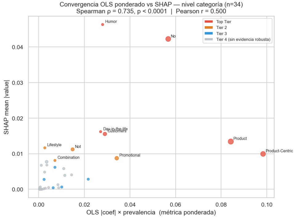
Figura 4.5: Convergencia entre OLS (coeficiente ponderado por prevalencia) y SHAP ( |\text{SHAP}| promedio) a nivel de categoría individual ( n = 34 ). La correlación de Spearman es \rho = 0,74 ( p < 0,001 ).
