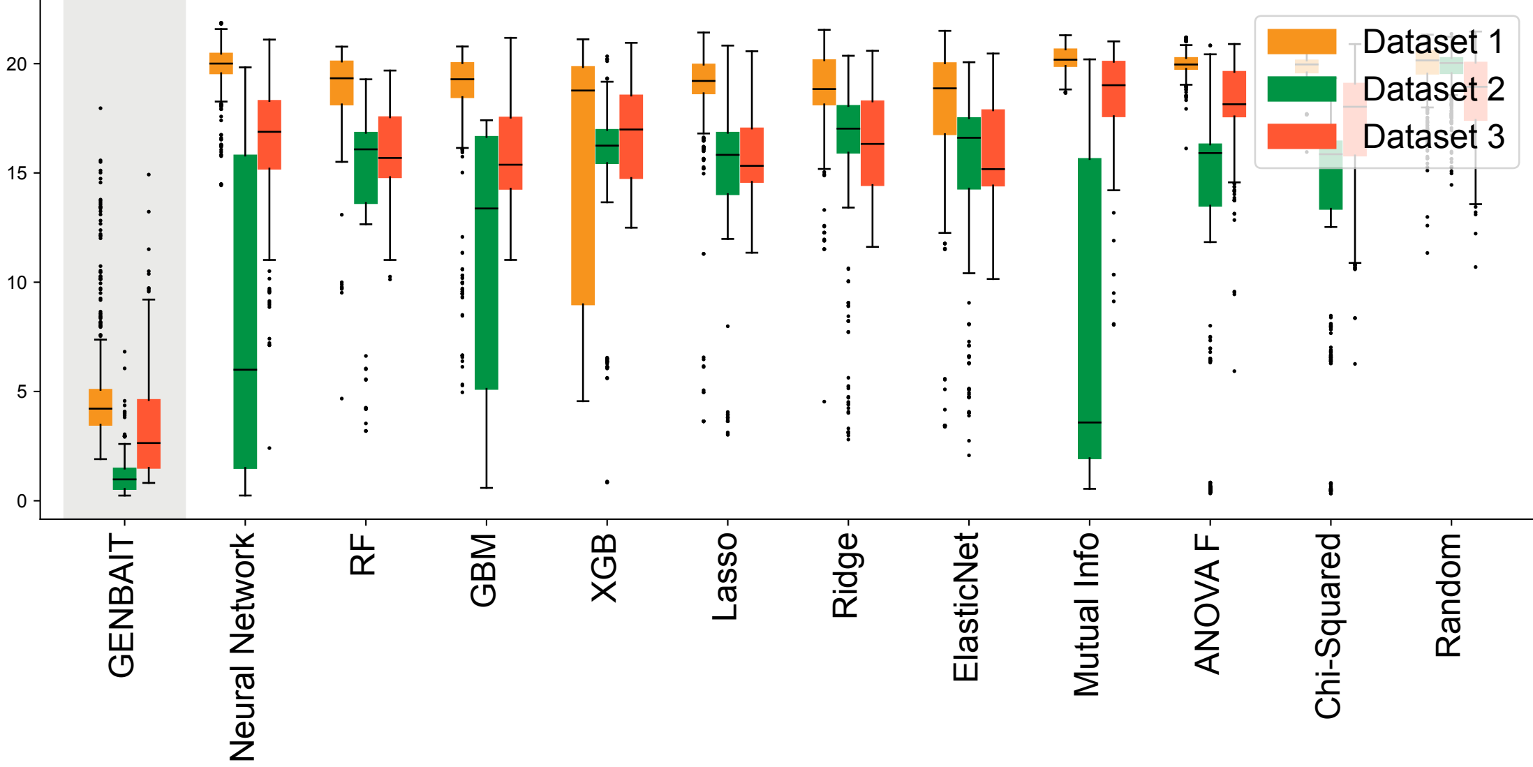
NMF min KL divergence score
