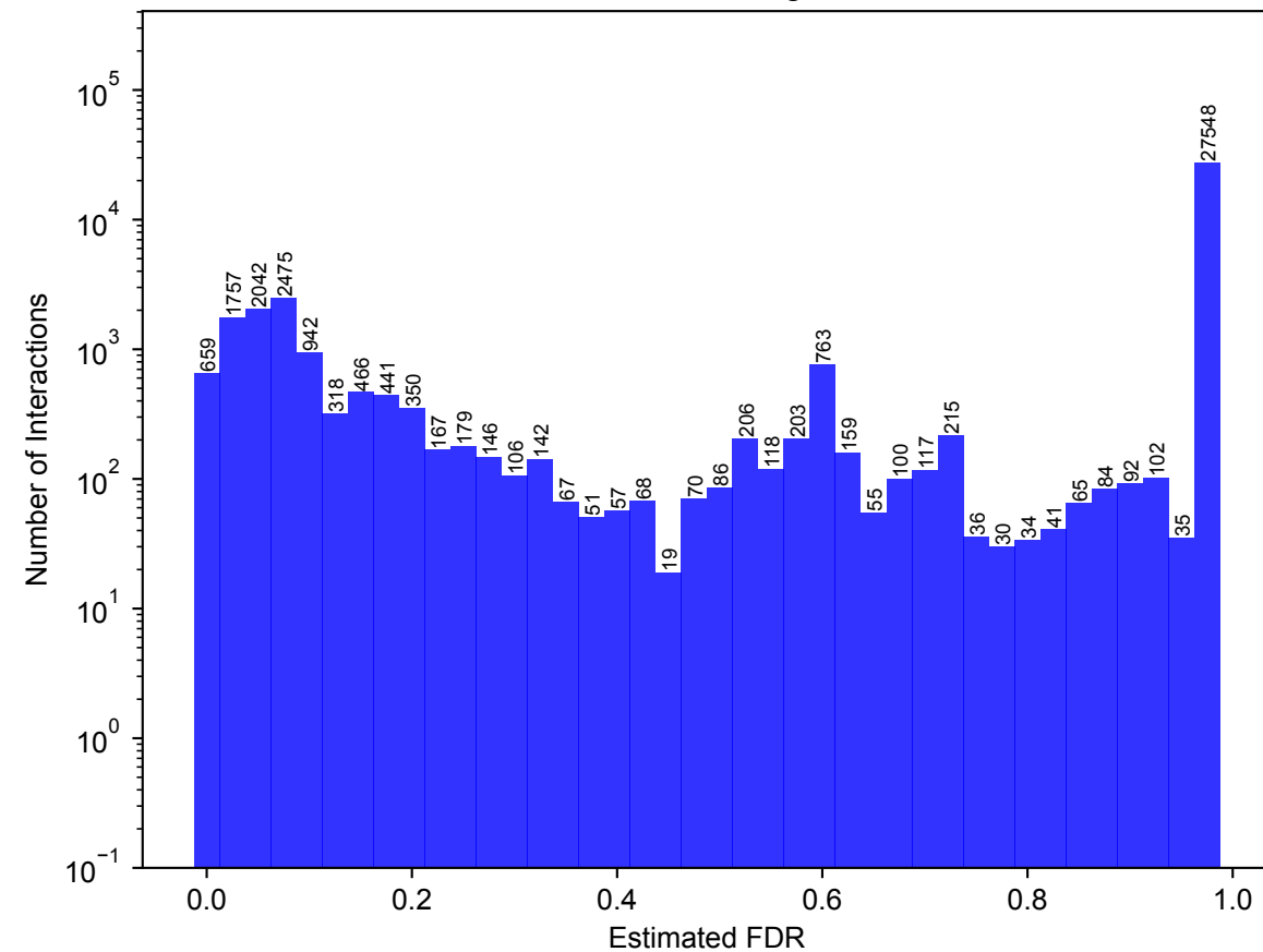
PU Learning
