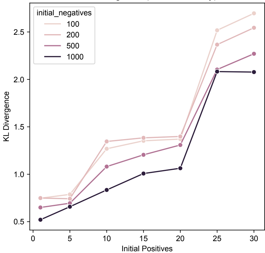
KL Divergence (Real vs Decoy)
