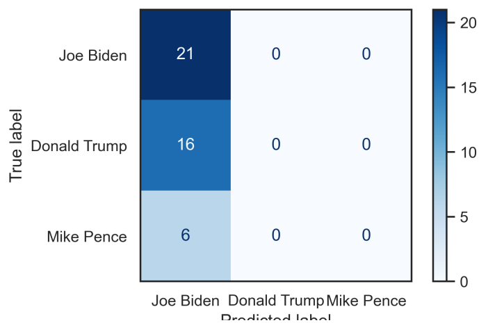
Figura 8: Matriz de Confusión Naive Bayes.
