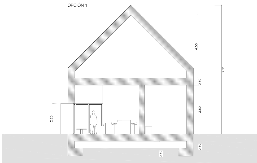
SECCIÓN A-A'
