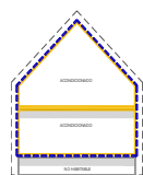
RELACIÓN DEL CAMBIO DE AIRE A 50 Pa [n 50 ]
