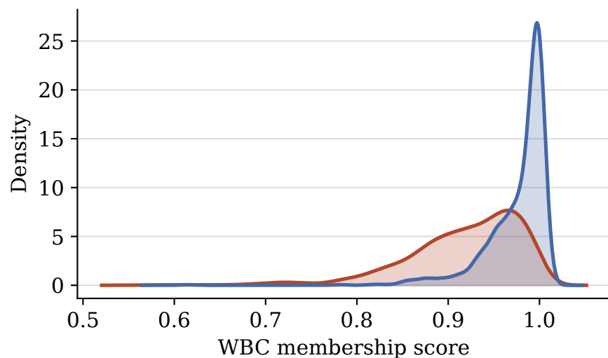
Llama-3.2-1B-IT WBC AUC=0.592
