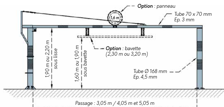
Partie centrale portique (2 vantaux)
