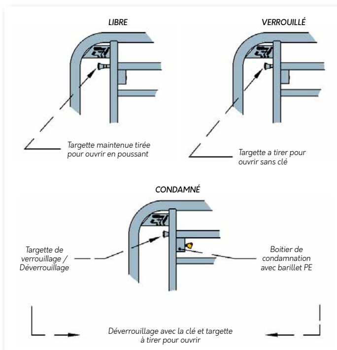
Sélecteur de fonctionnement (option)
