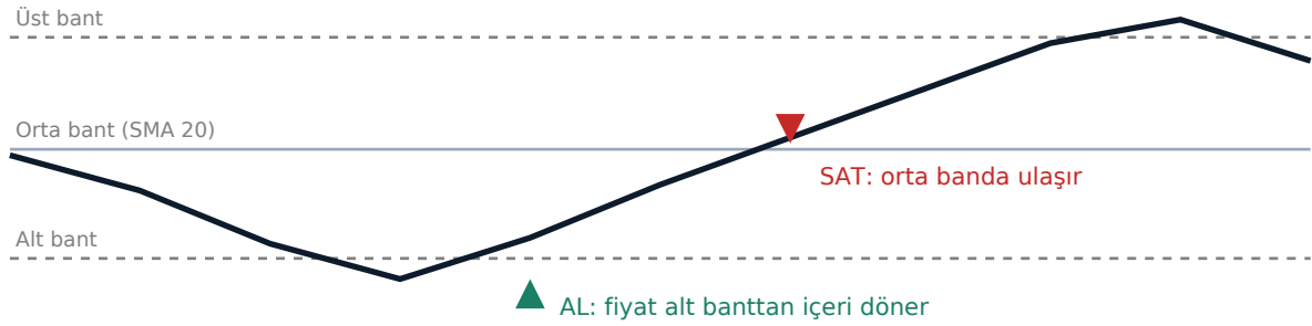
Şekil 2 — Ortalamaya dönüş mantığı (Bollinger / RSI).
