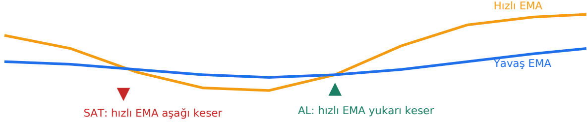
Şekil 1 — Trend takip mantığı (EMA kesişimi).
